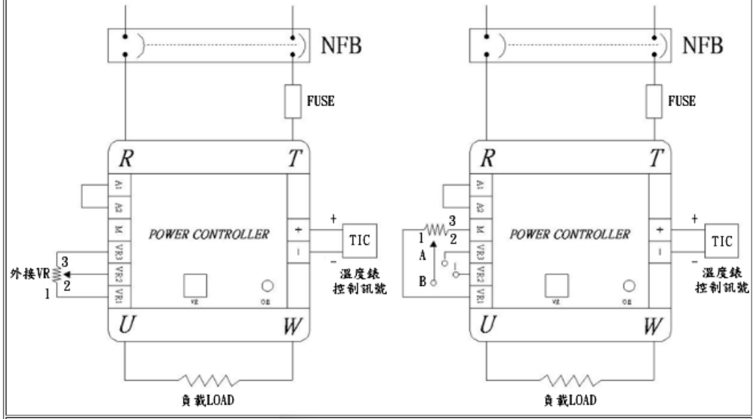
串接模式示意圖：(電流)
