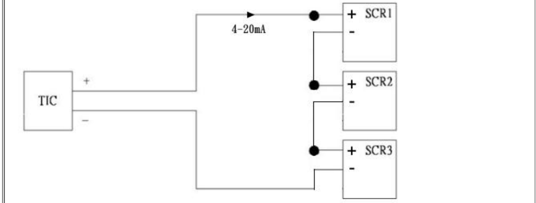
並接模式示意圖：(電壓)
