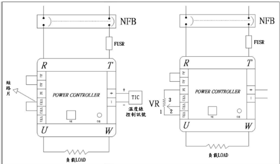
自動+外接VR(輸出功率限制)
