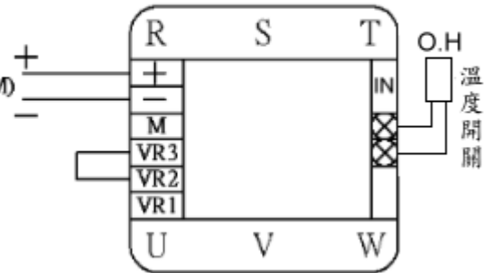
5.自動模式(P.W.M)
