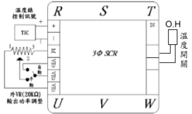
3.自動(4-20mA)+手動+外接開關模式
