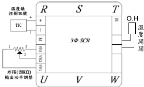
2.自動(4-20mA)+限制輸出量<->
